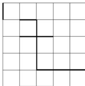
邊滲流
