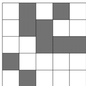
點滲流
